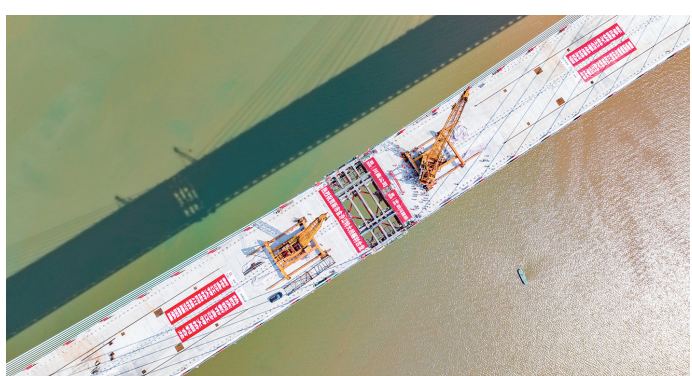
新市金沙江特大桥建设现场。
